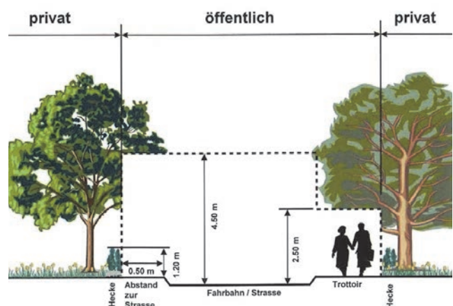
Lichtraumprofil bei Verkehrsflächen
